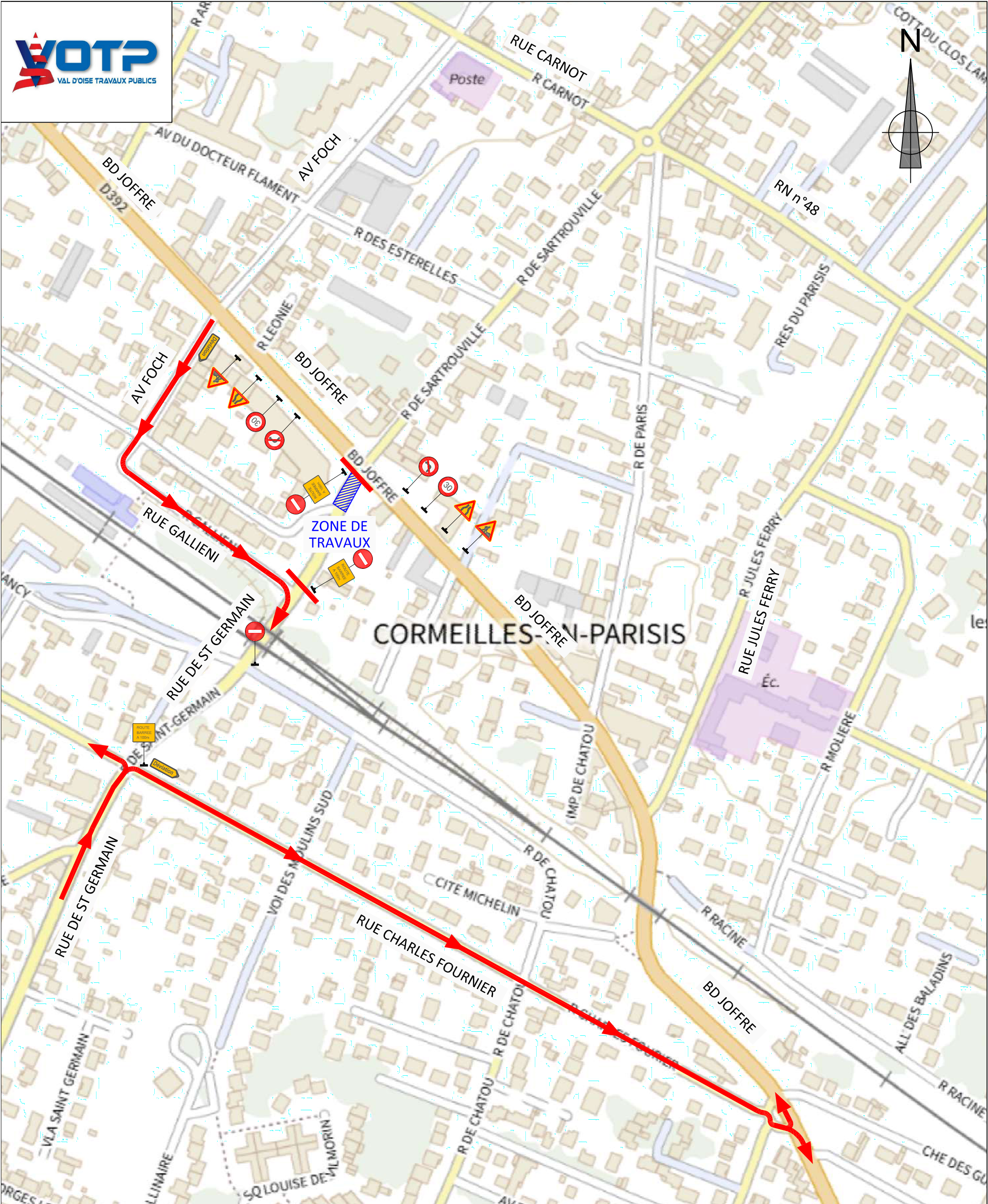
Commune de Cormeilles en Parisis TRAVAUX RUE DE SAINT GERMAIN Plan de circulation PHASE 2: du 20/07/2026 au 31/08/2026
